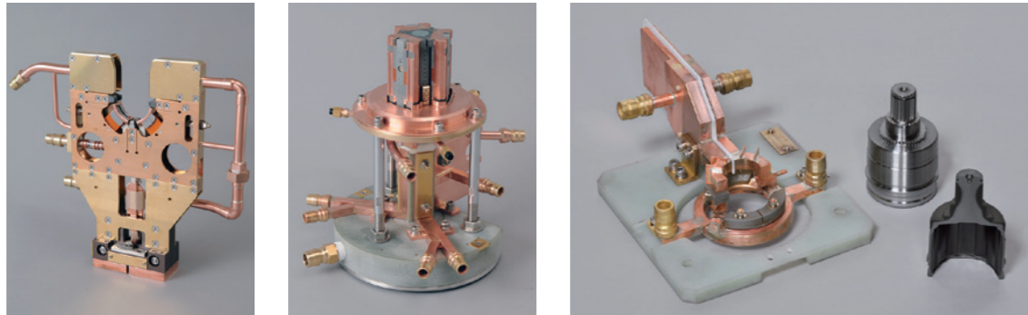
クランクシャフト焼入コイル インボード溝部一発焼入コイル CVJ軸部焼入コイル
