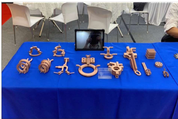
△3D プリントで製作した加熱コイル
