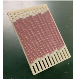
反射角可変反射板
