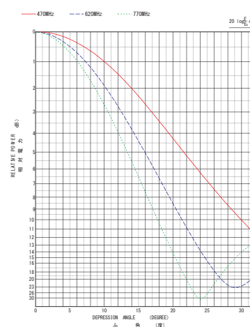
垂直面指向性図
